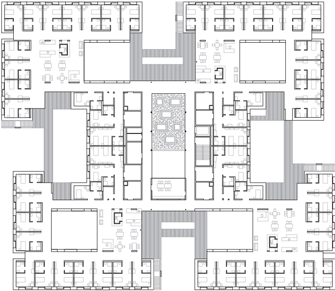
obergeschoss / first floor
